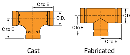
Fig. 7060 Tee
